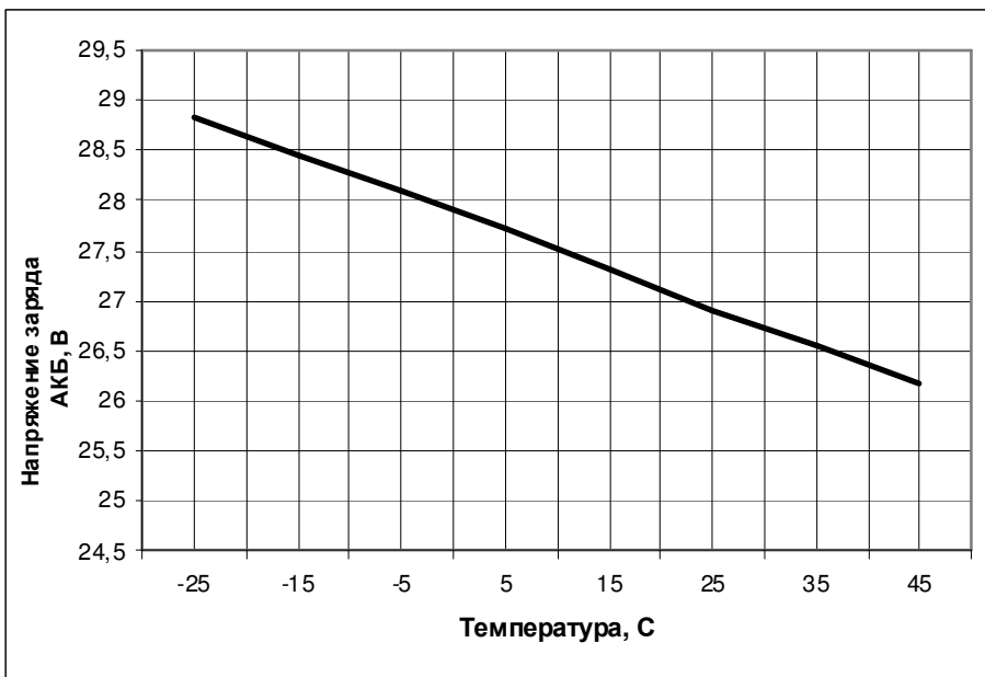
Рисунок 3 — Зависимость напряжения заряда АКБ от температуры
