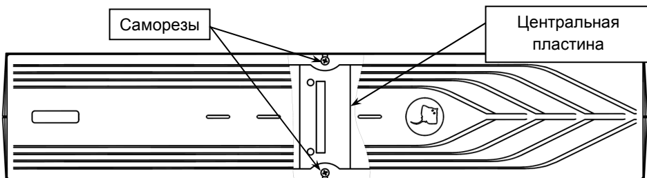
Рисунок 6 – Крепление центральной фиксирующей пластины
