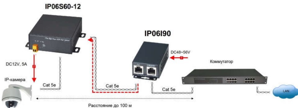
Рис.6 Схема подключения сплиттера IP06S60-12 и инжектора IP06I90 Рекомендации по монтажу и установке
