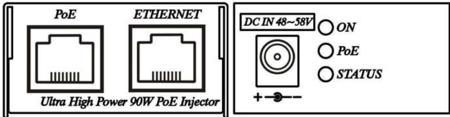
Рис.2 Разъемы и индикаторы IP06I90
