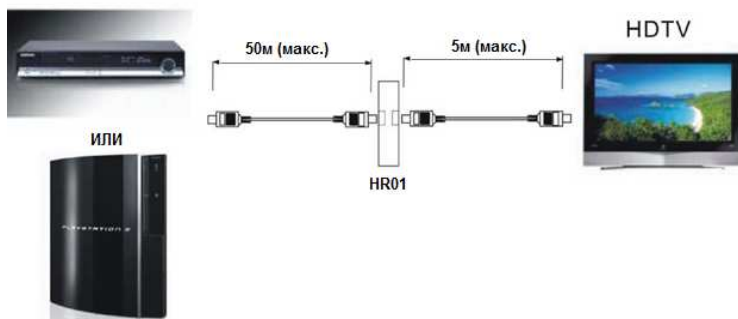
Рис.1 Схема подключения HR01
