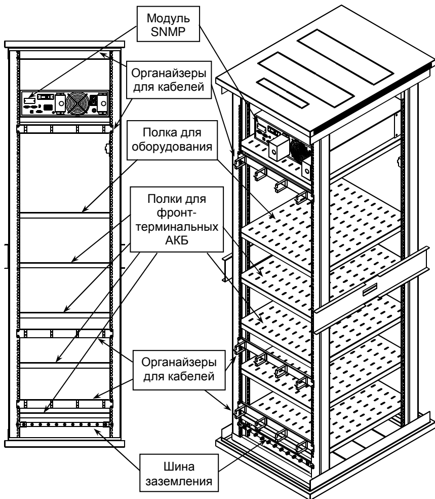
Рисунок 2 — Общий вид изделия сзади, без оболочки.
