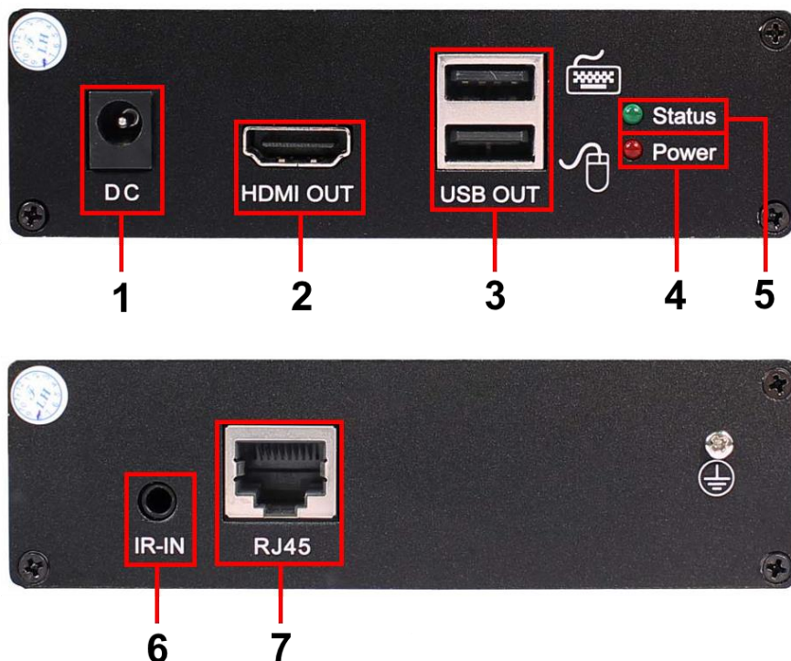
Рис. 3 Приемник RLN-NiKM/1, разъемы и индикаторы передней и задней панели
