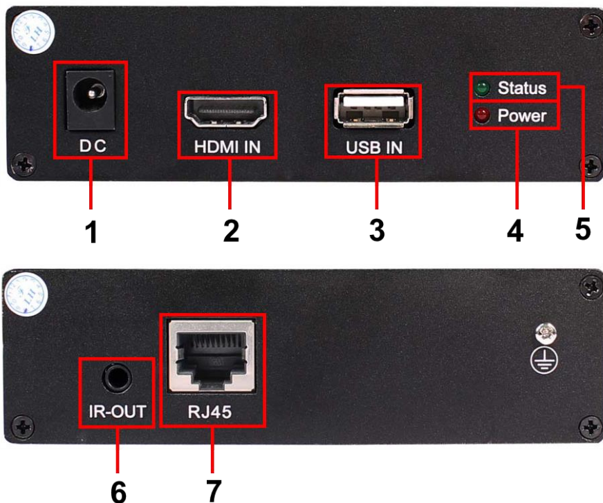
Рис. 2 Передатчик TLN-NiKM/1, разъемы и индикаторы передней и задней панели
