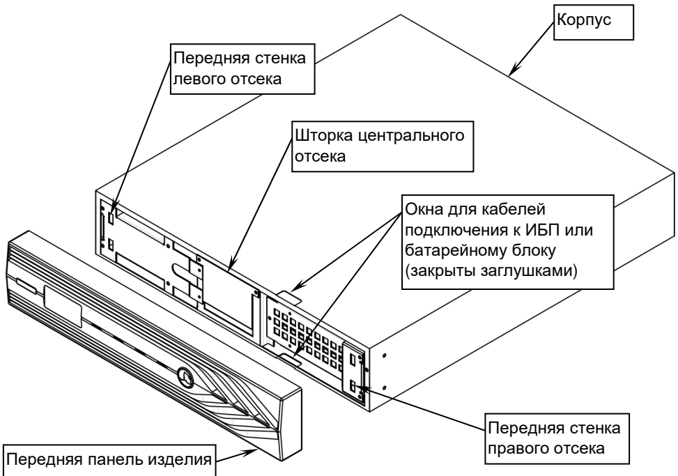
Рисунок 1 – Общий вид изделия со снятой передней панелью
