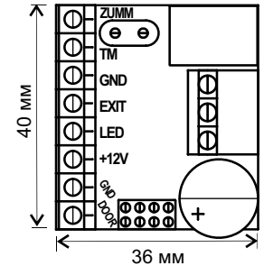
Рис.2 Внешний вид платы
