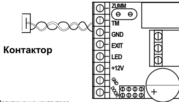
Рис. 5 Подключение контактора
