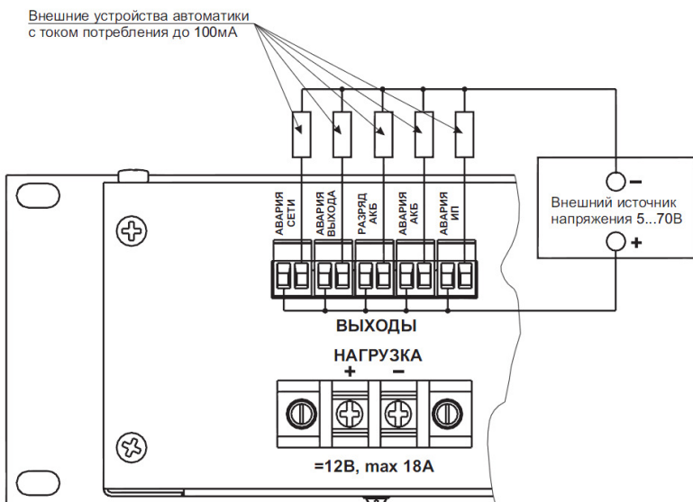
Рисунок 6 – Подключение внешних устройств автоматики.
