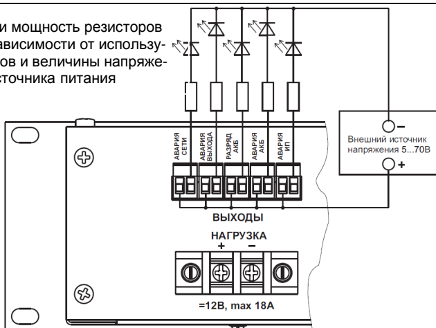
Рисунок 7 – Подключение внешних индикаторов
