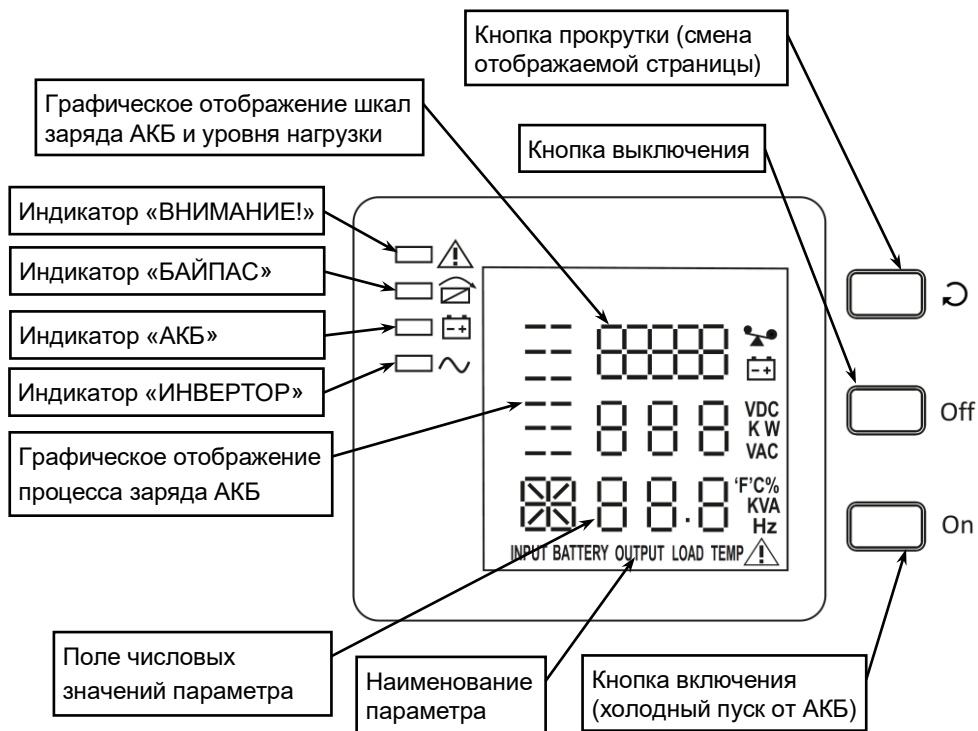
Рисунок 3 — ЖК-дисплей
