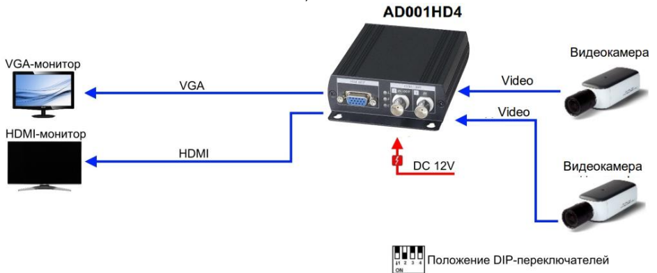
Рис.5 Схема подключения AD001HD4. Режим подключения 2-х источников видеосигнала.
